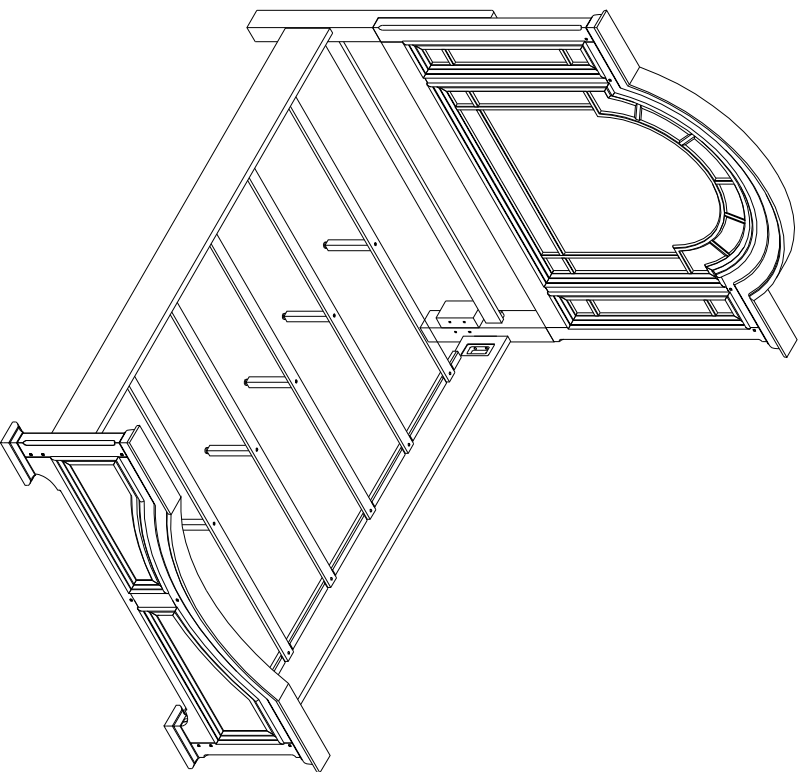
I x2 Allen bolt \phi 5/16" \times 38\text{mm} * x2 Vis à tête creuse hexagonale \phi 5/16" \times 38\text{mm} x2 Perno Allen \phi 5/16" \times 38\text{mm}
