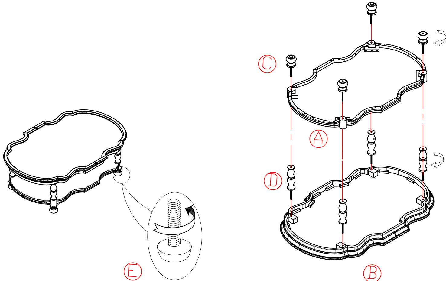
Adjustable leveler Patin réglable Nivelador ajustable
