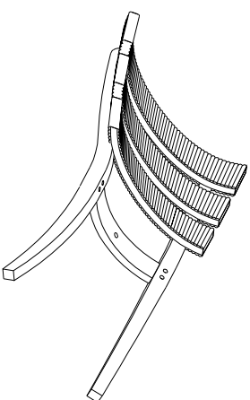
x1 RP361-260-BACK- Chair Back Dossier de chaise Pespaldo de silla *
