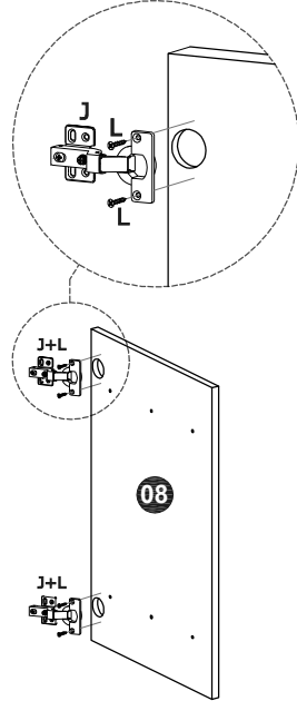
DETAIL 3 / DÉTAIL 3
