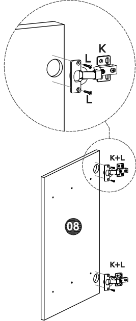
DETAIL 2 / DÉTAIL 2
